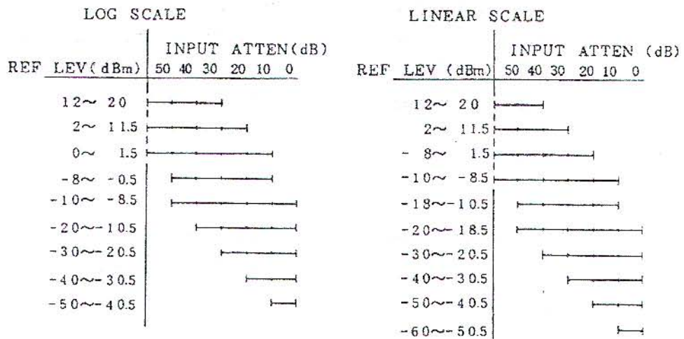
Fig. 5-4 INPUT ATTEN Range
