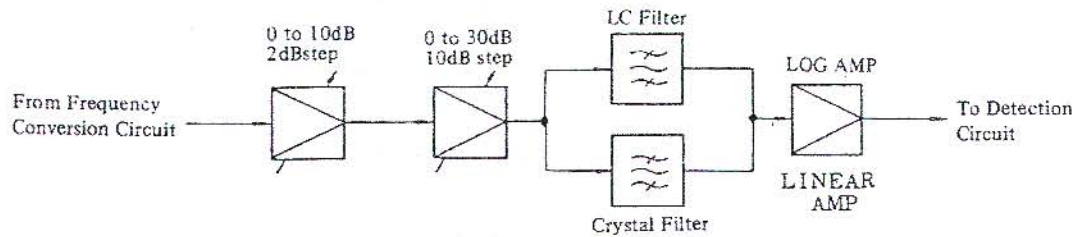
Fig. 3-3 MS610A IF Circuit
